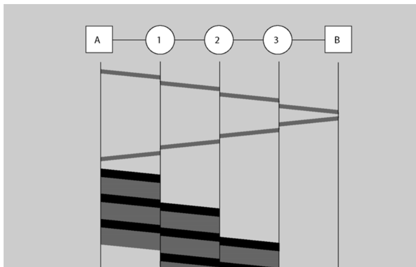
Figura 7. Diagrama temporal de una conexión en modo circuito virtual
