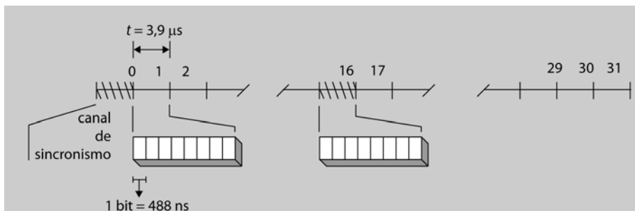
Figura 14. Representación de la trama E1
