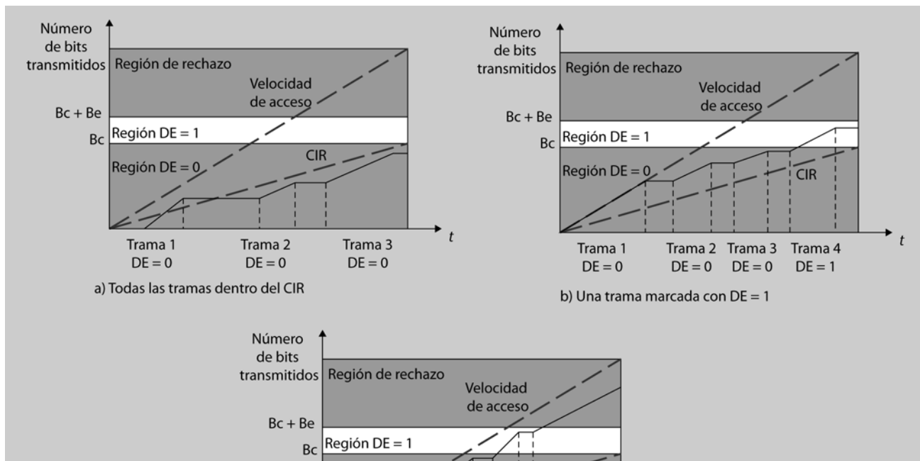
Figura 31. Ejemplos de gestión del tráfico
