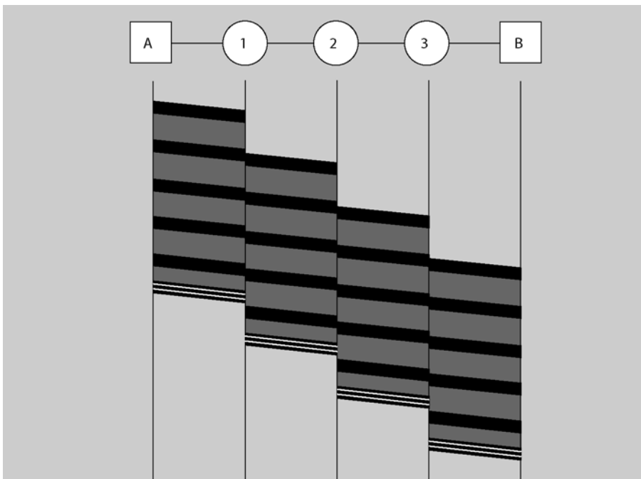
Figura 6. Diagrama temporal de una conexión en modo datagrama
