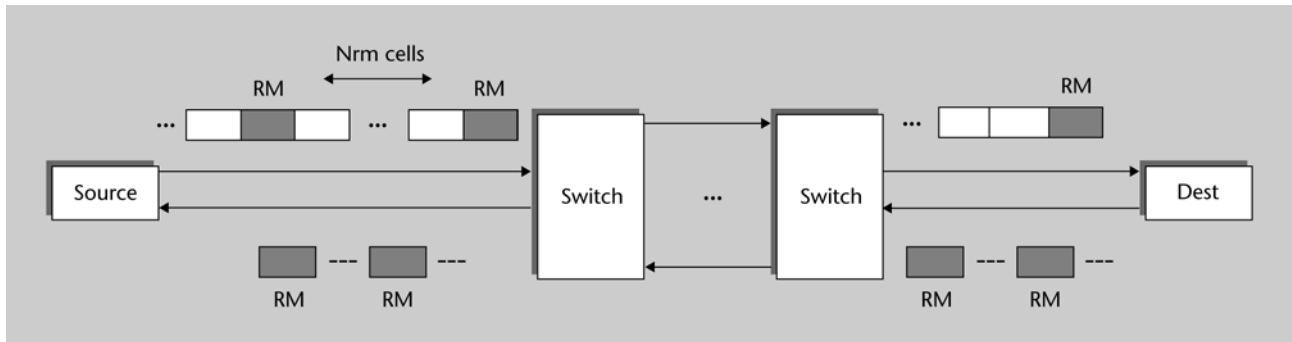
Figura 45. Mecanismo ABR
